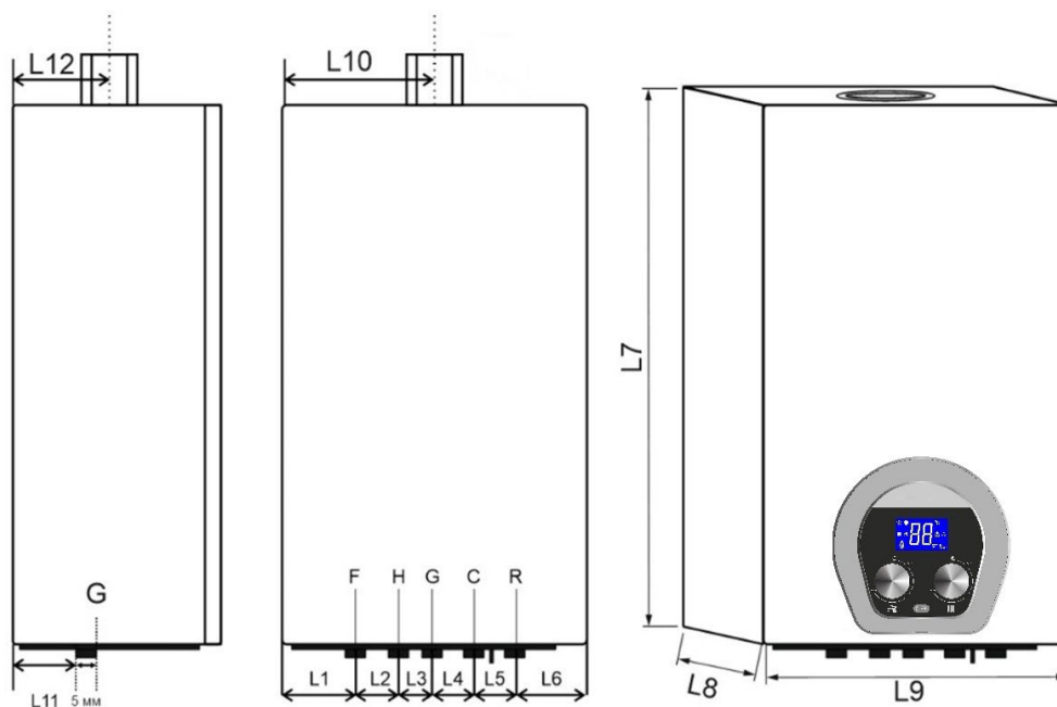
Рис.11 Габариты котла и его присоединения
