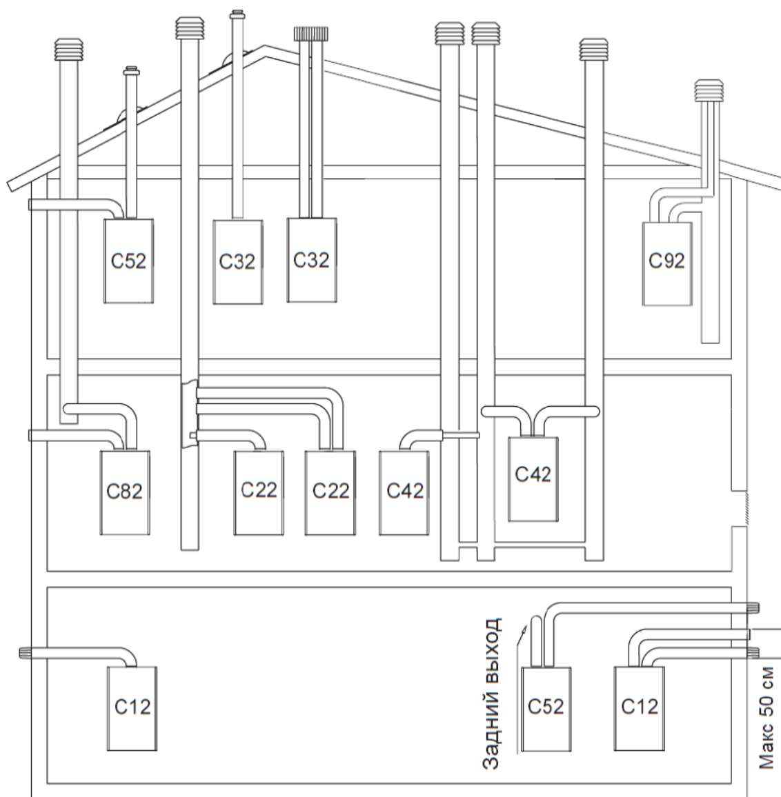
Рис.9 Дымоудаление типов С
