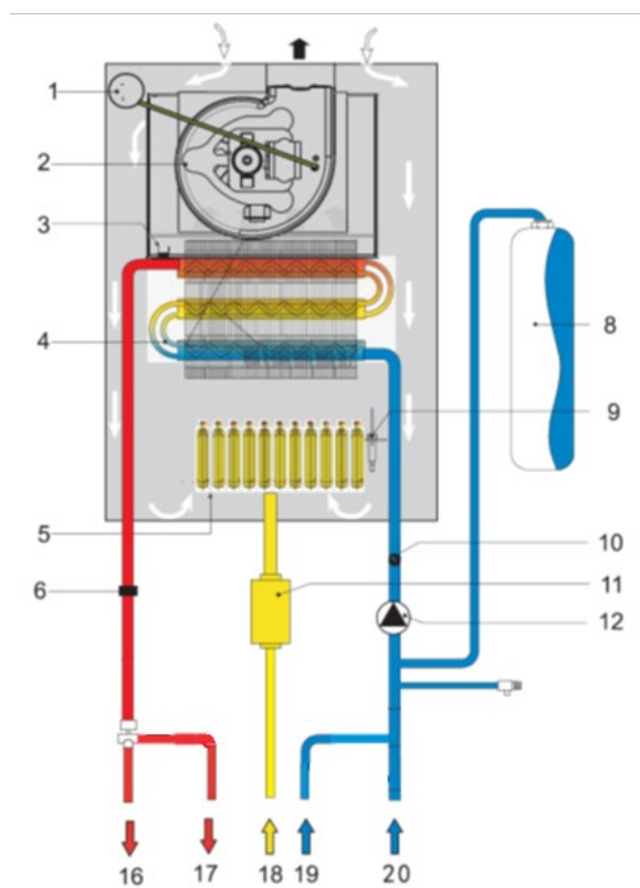
Рис.4 Принципиальная схема котла мощностью 24, 32 кВт
