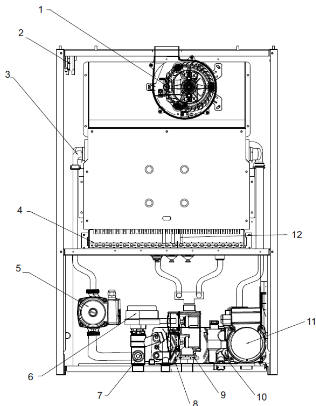
Рис.1 Конструкция котла мощностей 12-32кВт
