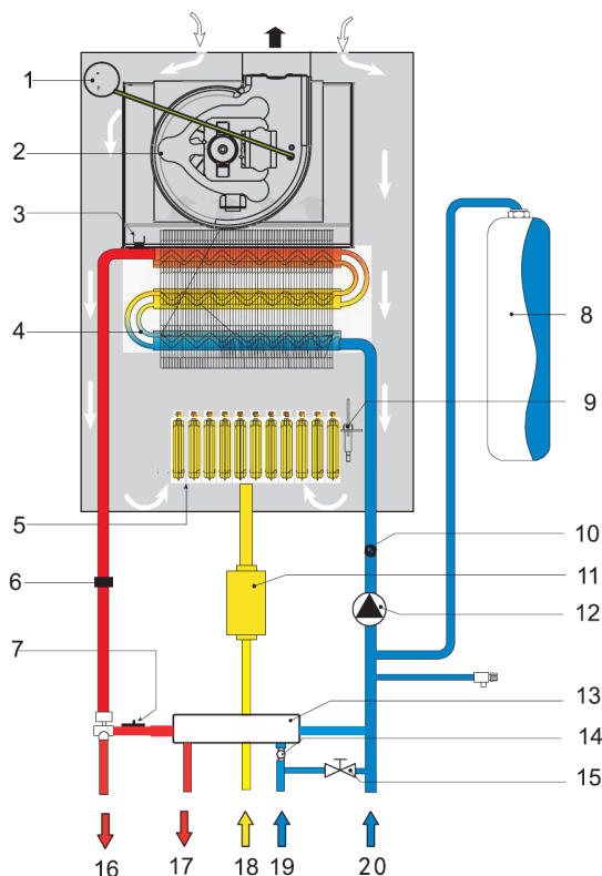
Рис.2 Конструкция котла мощностей 40-50кВт
