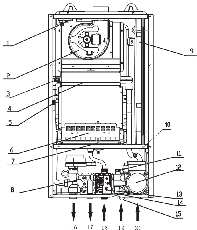
Рис.1 Конструкция котла мощностей 12-32кВт
