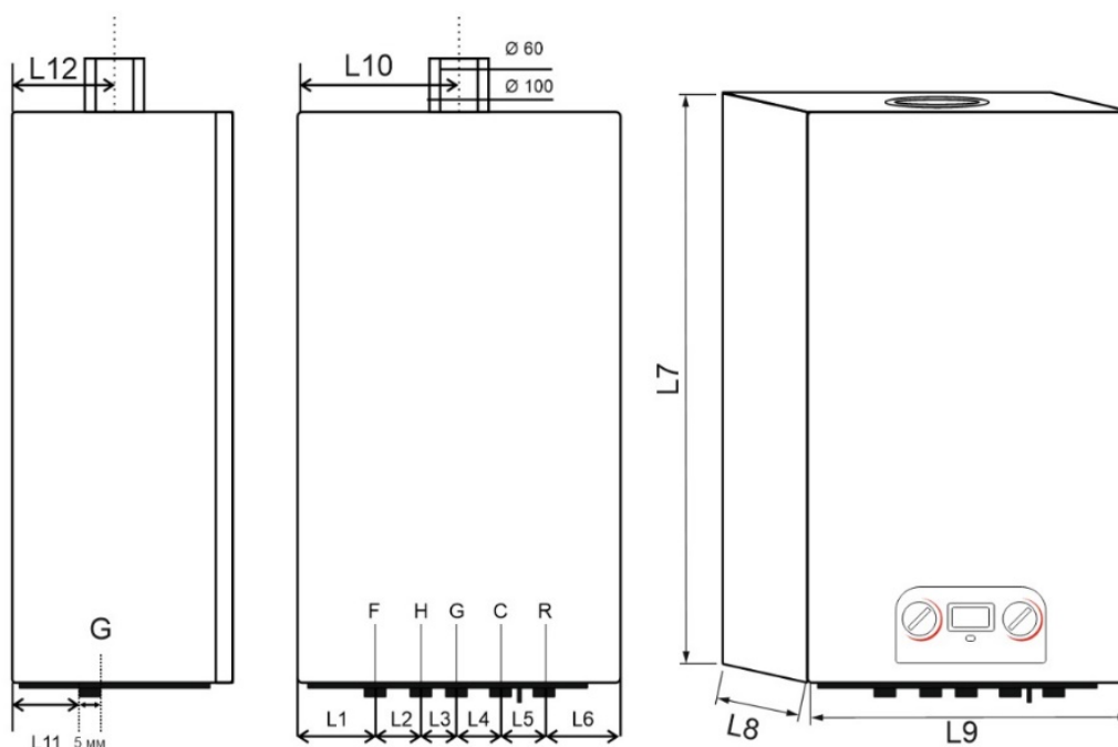
Рис. 7 Габариты котла и его присоединения
