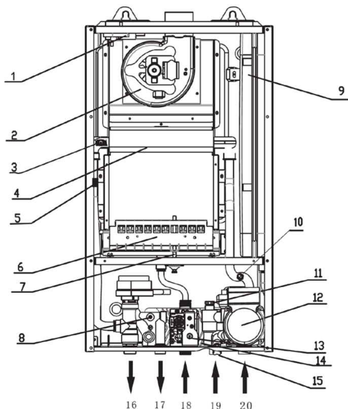
Рис.2 Конструкция котла
