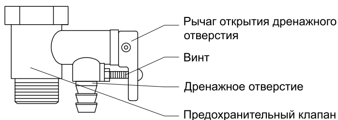
Рисунок 2. Предохранительный клапан.
